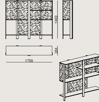
THRESHOLD DOLAP S0 H3L2 MELAMİN EPOKSİ Toplam Genişlik: 1799 mm" Toplam Derinlik: 367 mm" Toplam Yükseklik: 1469 mm"
